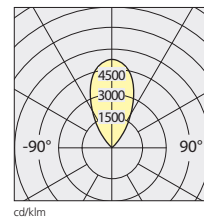
27W 4000 K α=6°x54°
